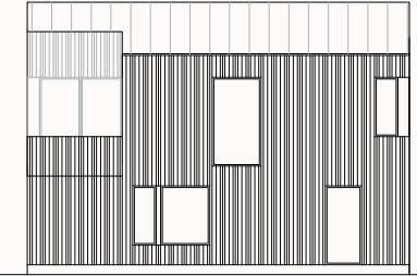
FASAD SÖDER
